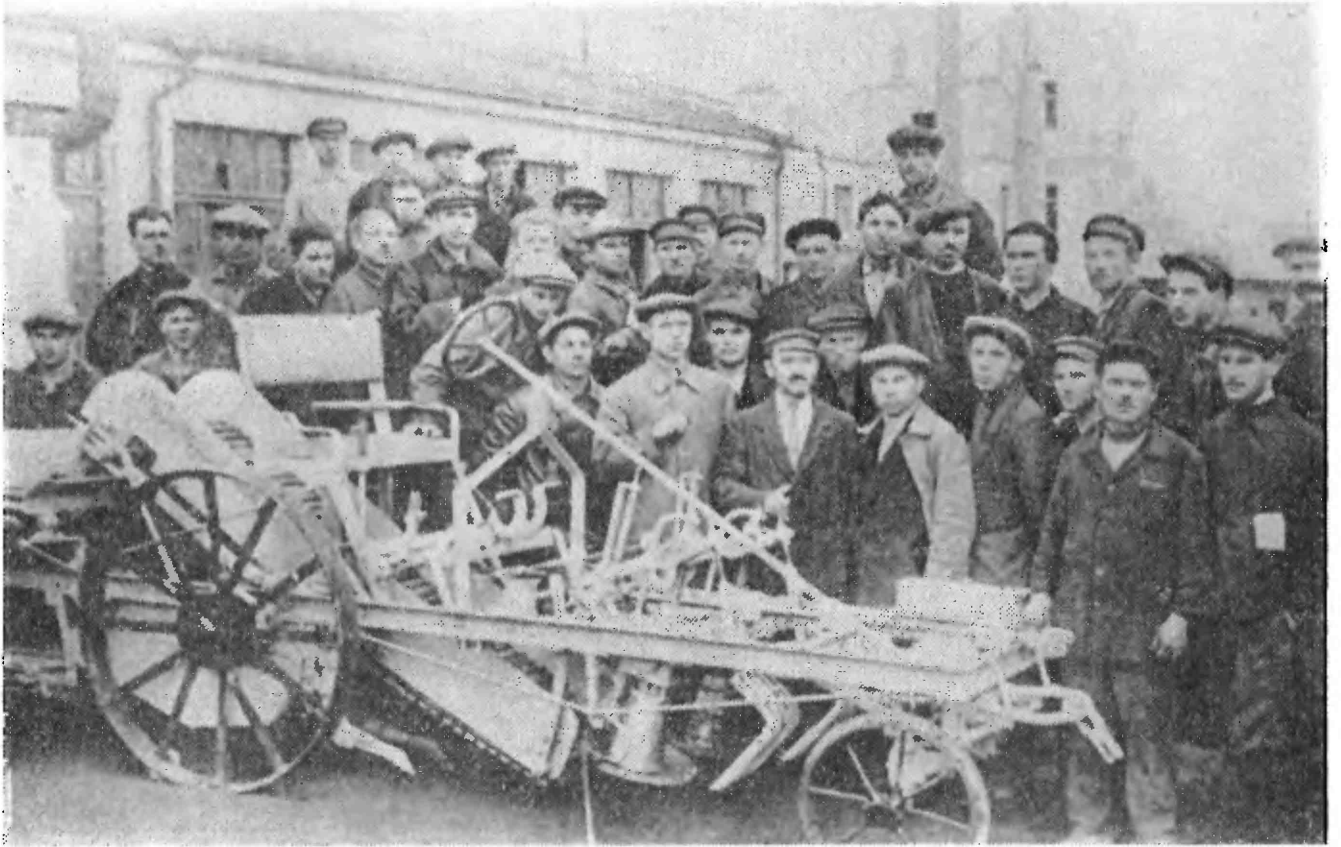
Первый свеклоуборочный комбайн, построенный в Николаеве на заводе «Плуг и Молот» в годы первой пятилетки
