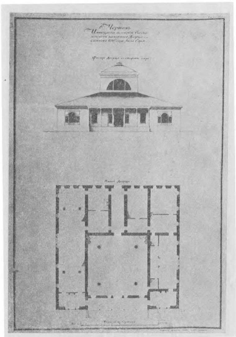
Дом Г. А. Потемкина в Богоявленске. 1790 г. Арх. И. Е. Старов Чертеж середины 1790-х годов
