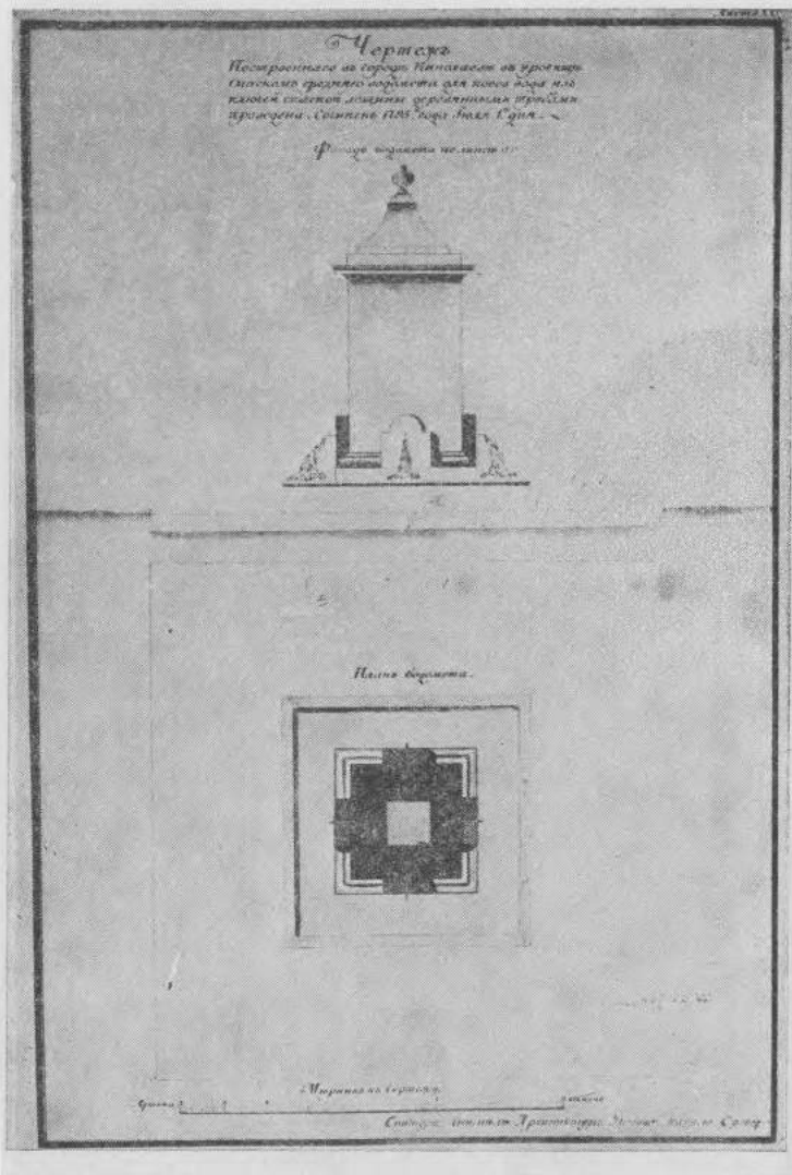
«Чертеж построеннаго в городе Николаеве в урочище Спаском средняго водомета для кою вода из ключей спаской долины деревянными трубами проведена. Соинен 1795 года. Июля 1-го дня» (публикуется впервые)
